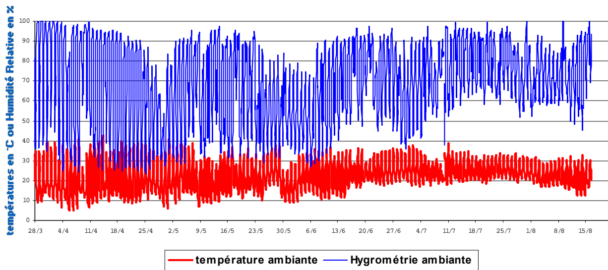
Graphique 1 : températures et hygrométrie ambiantes
