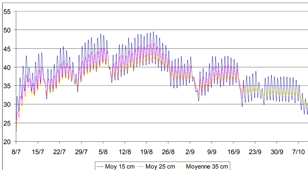
Graphique 2 : Températures du sol à 15, 25, 35 cm de profondeur – Solarisation 2011
